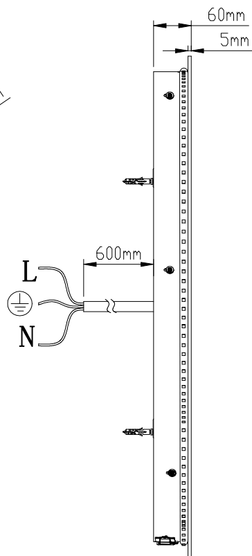
LEFT SIDE
