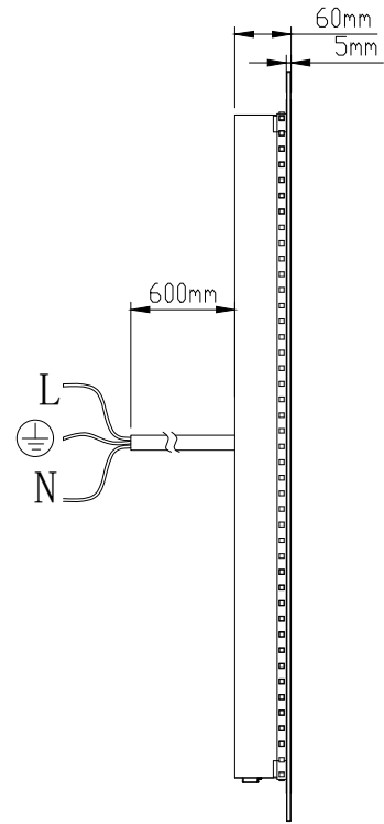
LEFT SIDE
